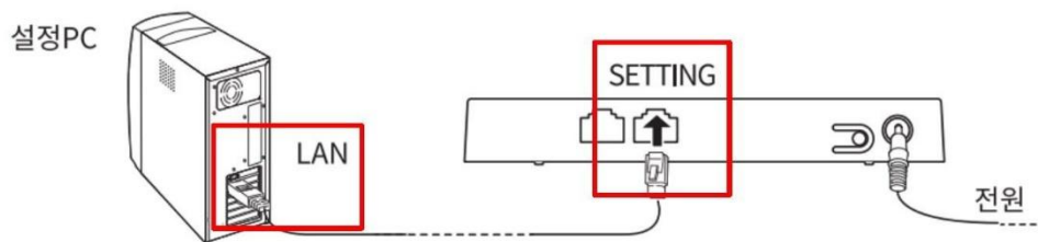
설정PC, RemoteWOL2 본체의 구성도
